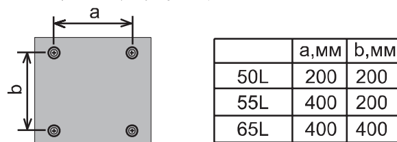
Рисунок 4 – Размеры для выбора настенного кронштейна
