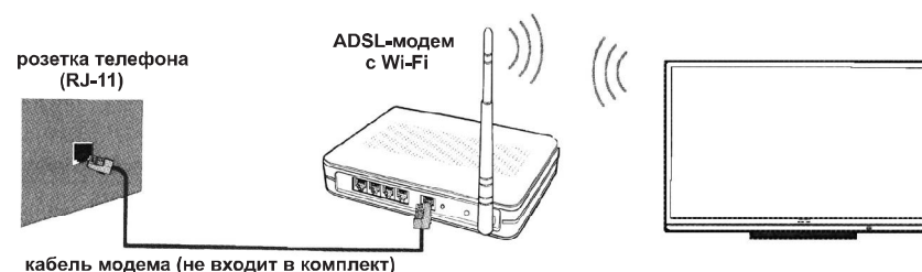
Рисунок 7 – Беспроводное подключение
